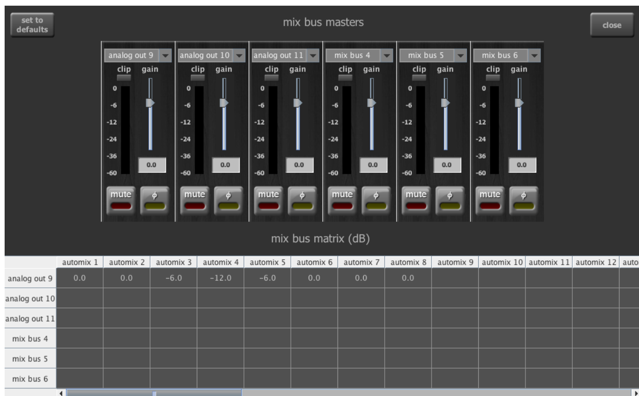
Figure 6-12 Dugan Control Panel のミックスバス・マトリックススクリーン
