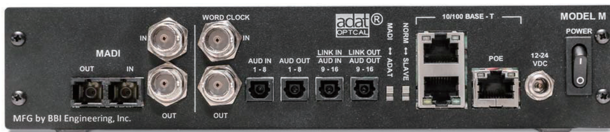
Figure 3-1 Model M リアパネルコネクタ
