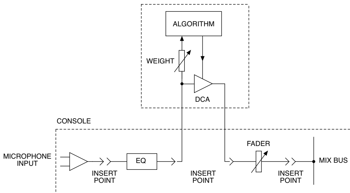
Figure 6-1 |一般的なアナログミキサーのプリフェーダーインサートポイント
