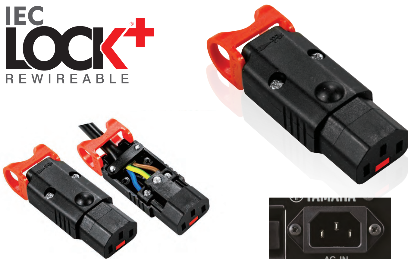
IEC規格 (C13) インレット
